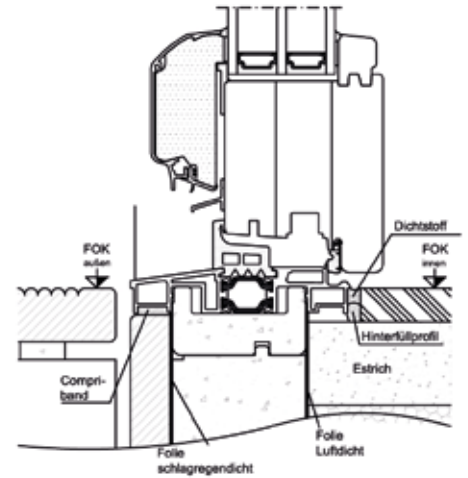
Bauanschluss mit Purenprofil unten
