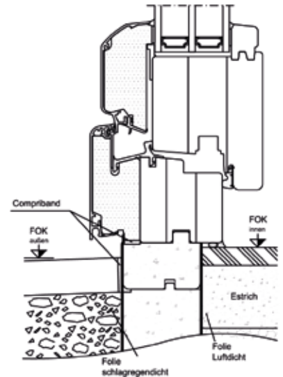
Bauanschluss mit Purenprofil unten
